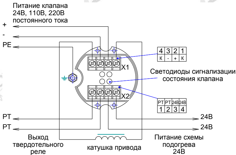
Рис. 6б Модуль-СФУ-12/24В, 110/220В постоянного тока. Схема подключения
