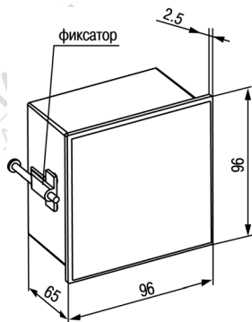
Рисунок 4.4 – Габаритные размеры корпуса Щ1
