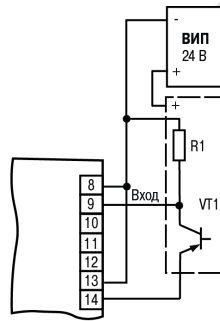
Рисунок 5.4 – Подключение датчиков с р-п-р-выходом: 1) пассивных; 2) активных
