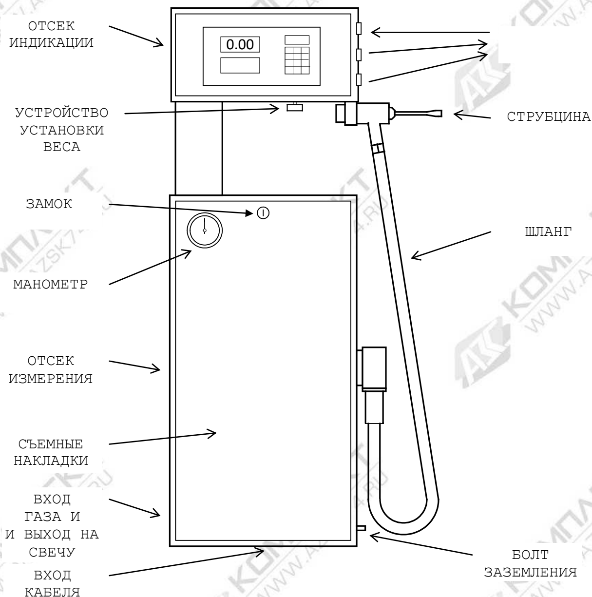
Рис.4 Пост наполнения
