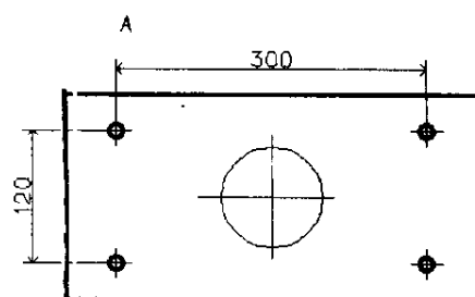
Рис.1 Установка УНСГ-01
