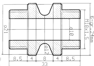
Рис.12 Разрывная вставка
