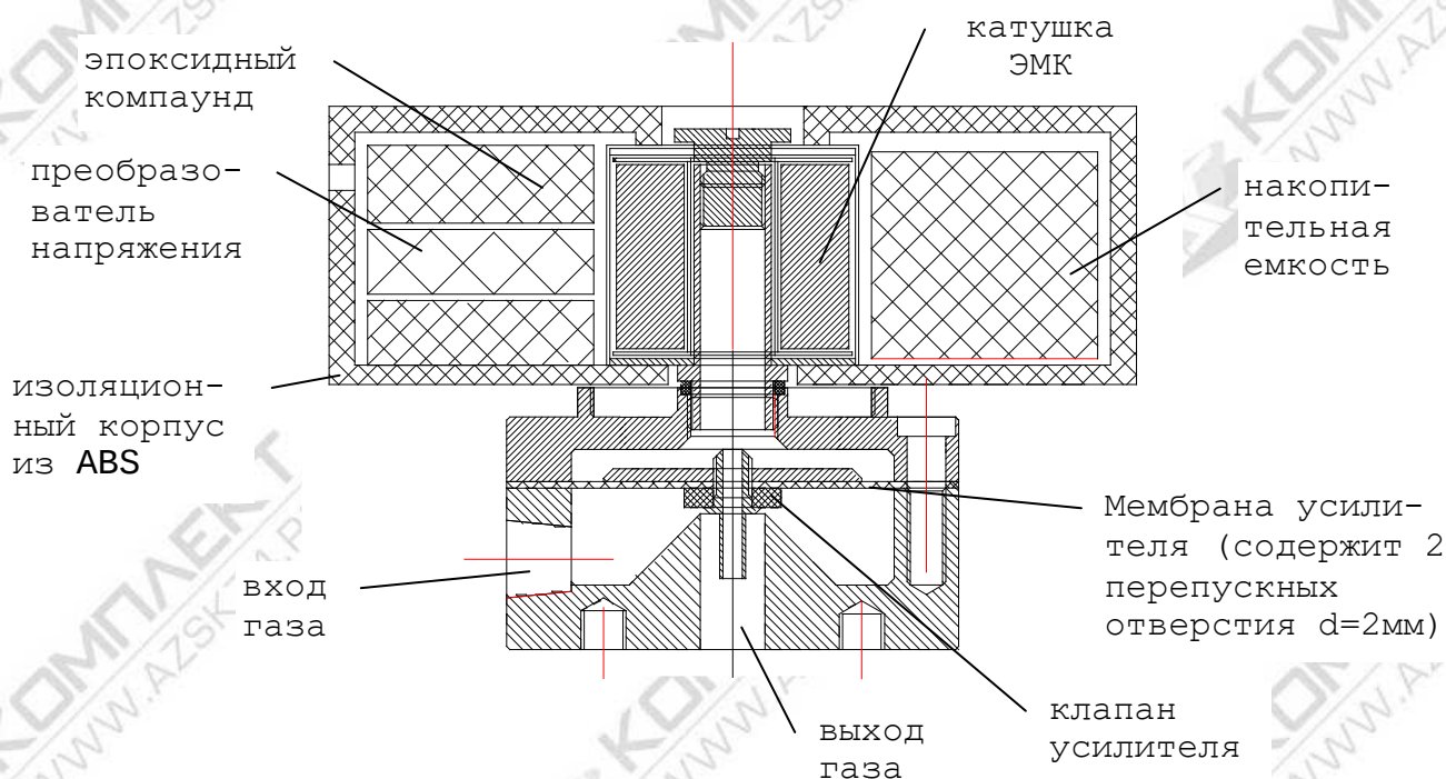
Рис.9 Электромагнитный клапан
