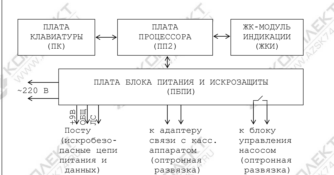
Рис. 3 Электрическая структурная схема пульта управления
