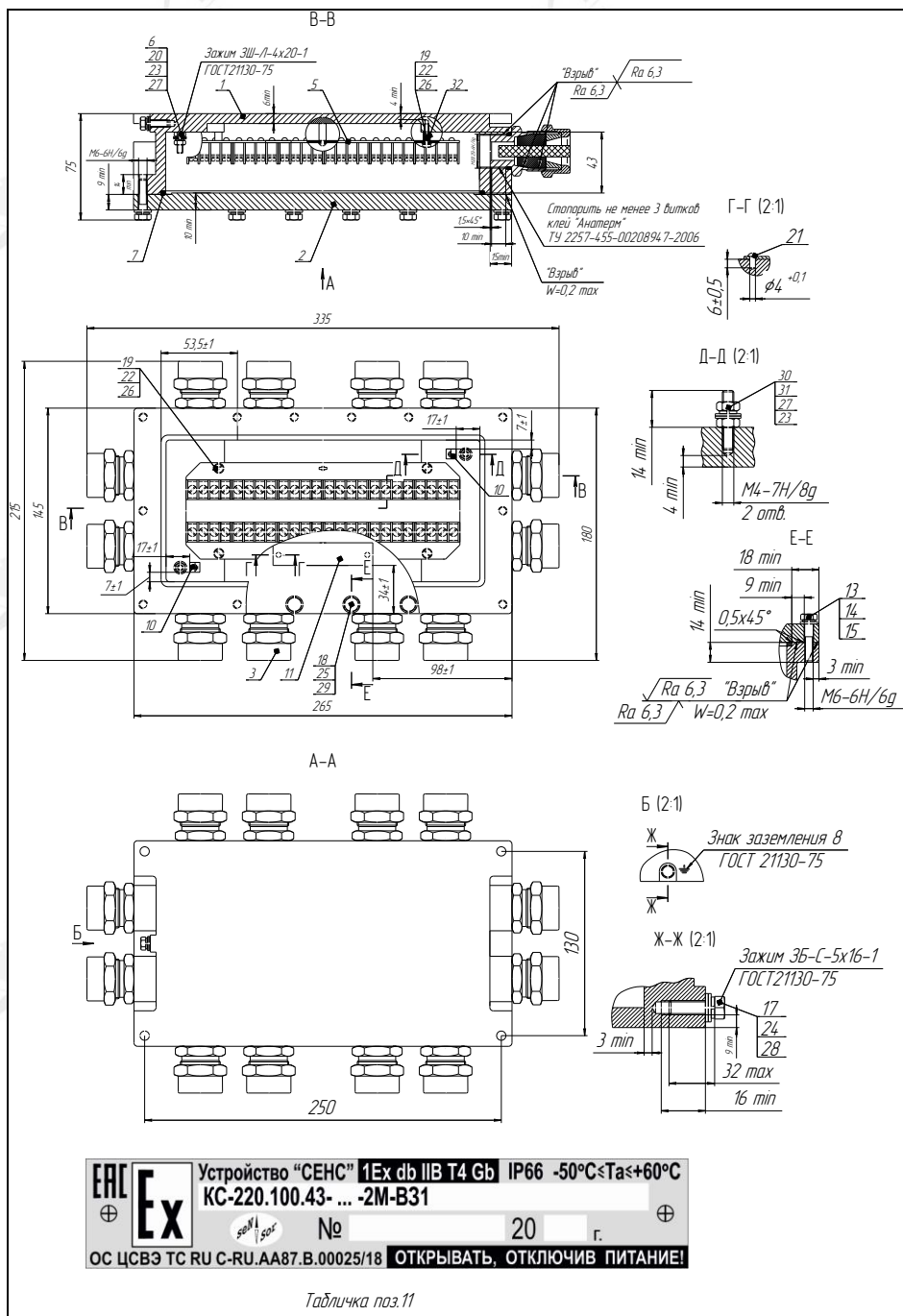
Рисунок. Б.1 – Чертеж средств взрывозащиты КС
