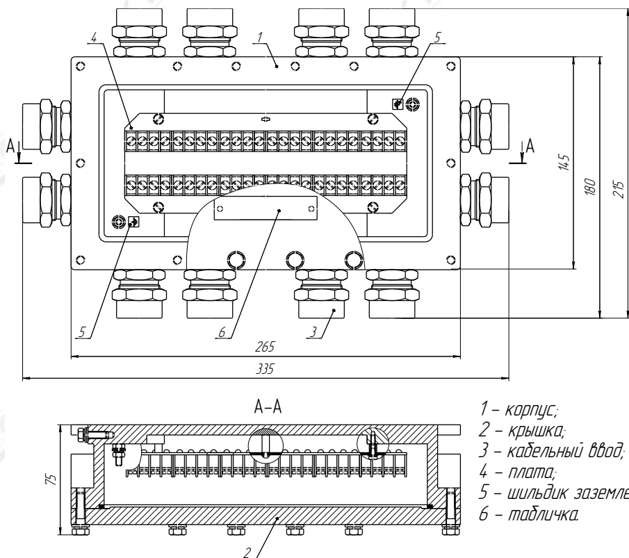
Рисунок 1 – Внешний вид (расположение кабельных вводов показано условно)
