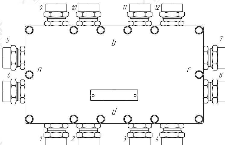
Рисунок 2 – Схема расположения кабельных вводов
