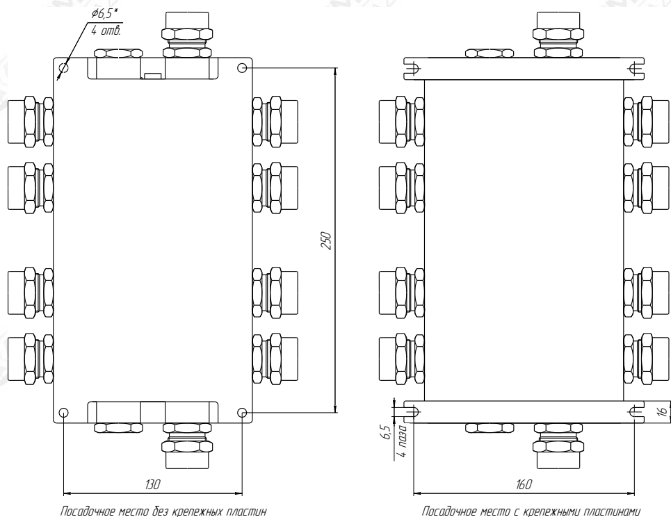
Рисунок 5 – Вариант крепления КС при помощи крепежных пластин
