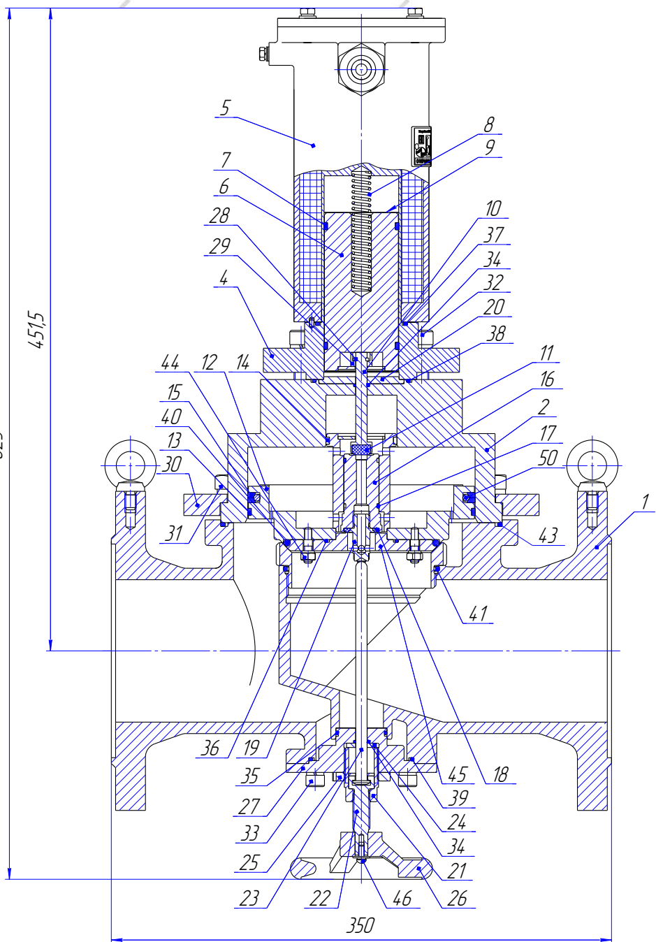
Рисунок 1а – Клапан СЕНС-ПР DN100PN25. Общий вид
