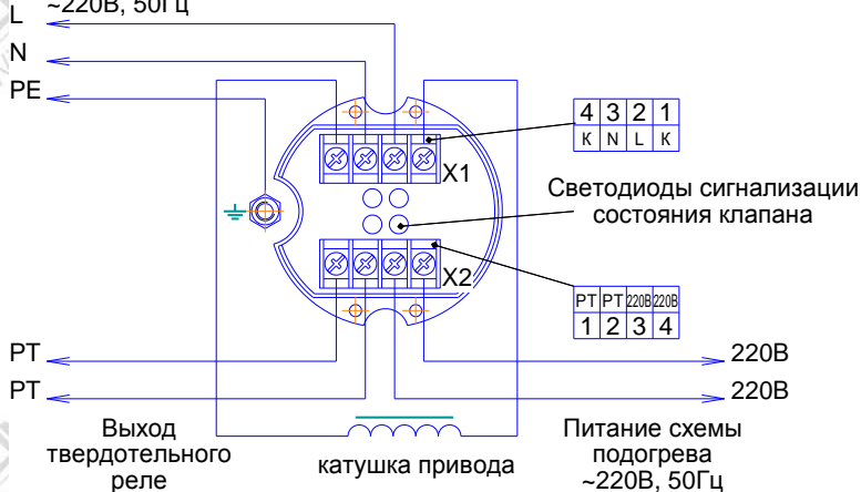
Рис. 7а Модуль-СФУ-220В. Схема подключения
