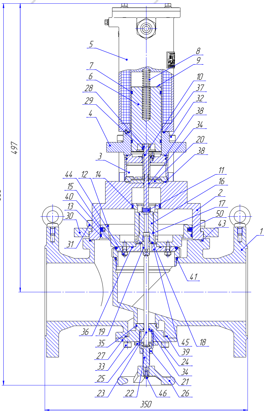
Рисунок 16 – Клапан СЕНС-ПР DN100PN25-ДКП. Общий вид
